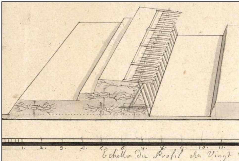
Figure 29 Profil de la terrasse d'un bastion. Détail du « Plan et Élévations de la ville de Québec » (Archives nationales d'outre-mer (ANOM), FR CAOM 3DFC434B)
