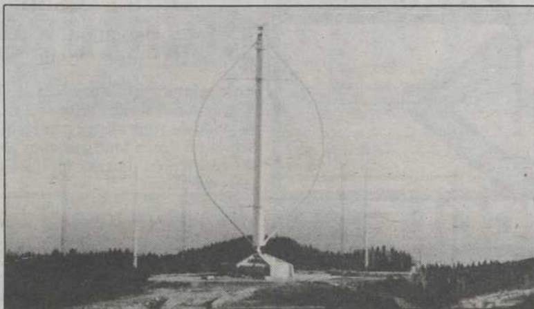
«Eole», l'installation de Cap-Chat est le rotor le plus puissant jamais construit avec sa capacité de 4 mégawatts suffisante pour alimenter 400 maisons.
