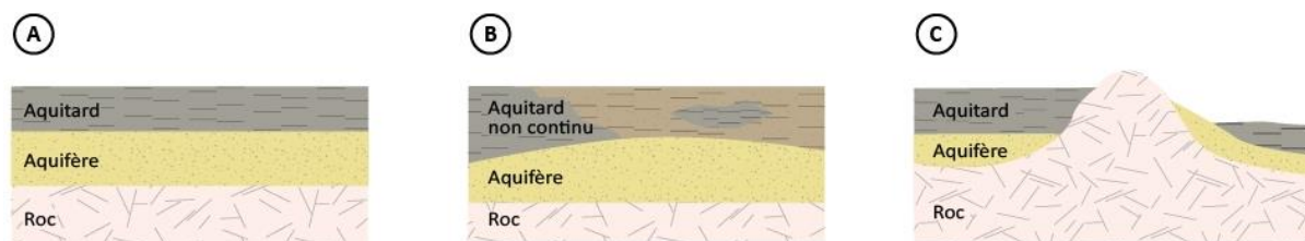
Figure 7 : Continuité des conditions de confinement : A) aquitard épais et continu sur toute l'aire d'alimentation; B) aquitard non continu constitué par exemple de dépôts alluvionnaires, deltaïques ou glaciaires, ou présence de lentilles d'argile; C) aquitard non continu avec affleurement rocheux par endroit
