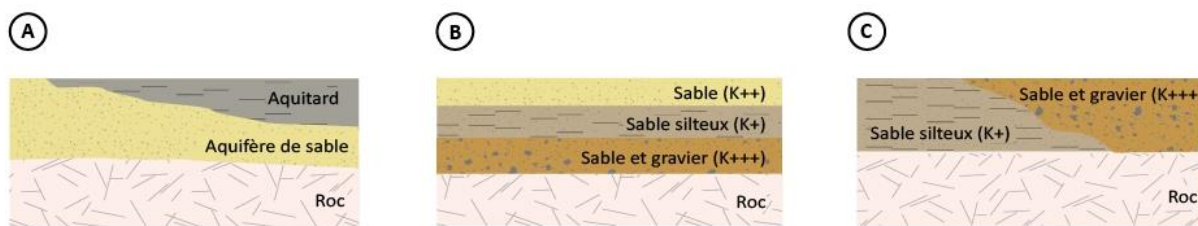
Figure 9 : Trois types d'hétérogénéité de l'aquifère : A) variation de l'épaisseur de l'aquifère qui fait varier sa transmissivité; B) aquifère multicouche aux conductivités hydrauliques différentes; C) changement latéral de conductivité hydraulique de l'aquifère
