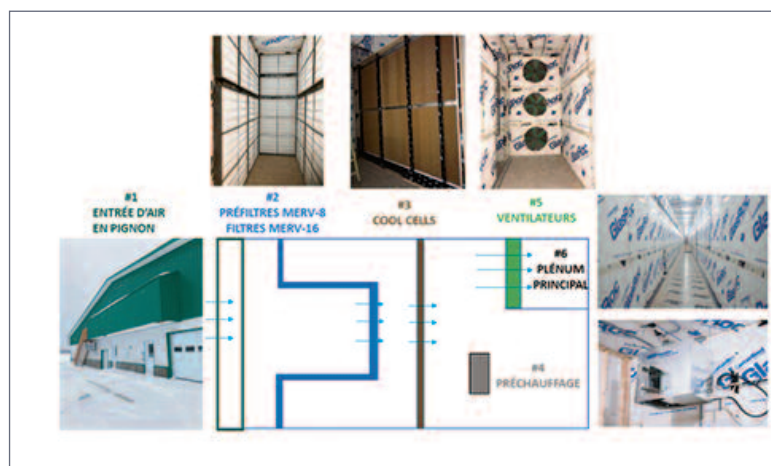
Figure 3 : Éléments du système de conditionnement de l'air d'une salle de traitement de l'air.
