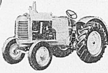
Massey-Harris "Bi-Force" "202". Un gros et fort tracteur, pouvant tirer 5 charrues, avec engin à 6 cylindres, quatre vitesses d'avant. Le démarreur automatique et l'allumage par batterie sont l'équipement régulier. "Bi-Force", une caractéristique exclusive Massey-Harris, donne du pouvoir additionnel pour les travaux sur la courroie. Les roues d'acier sont l'équipement régulier. Des pneus peuvent être obtenus sur demande spéciale.
