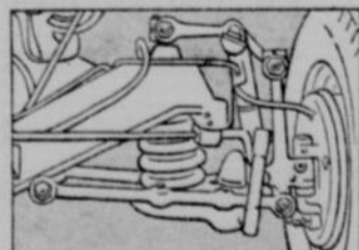
La suspension indépendante la plus perfectionnée donne à Plymouth son fameux roulement.
