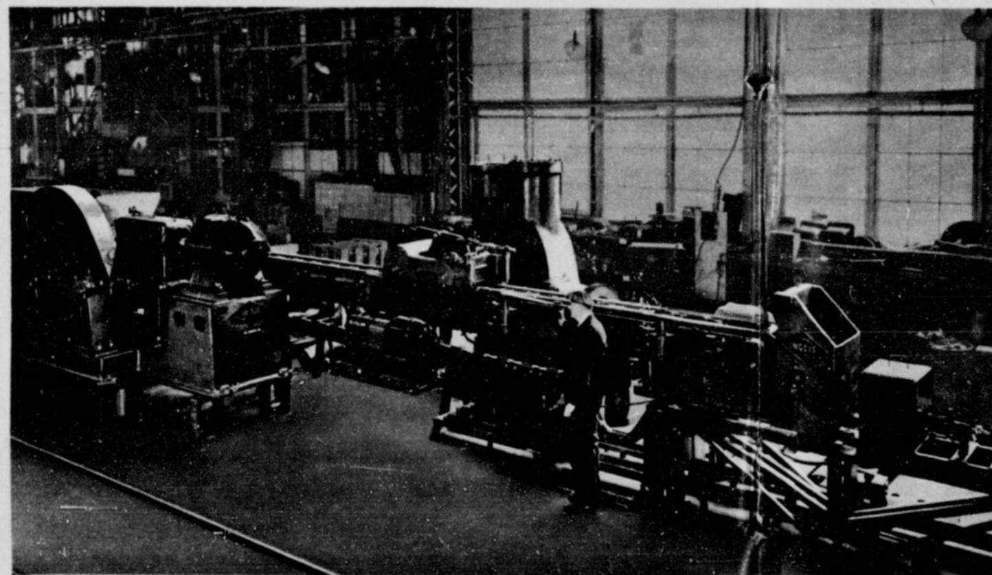
MAIS CE N'EST PAS DU CAMEL — c'est de l'acier roulé pur auquel on donne la forme désirée. Le génie mécanique INGLIS produit ce Banc à Tirer de 50,000 livres. Cet exemple intéressant de l'ingéniosité humaine étend l'acier pur avec la facilité et la nonchalance de la ménagère tirant le fil à travers le chas d'une aiguille.
