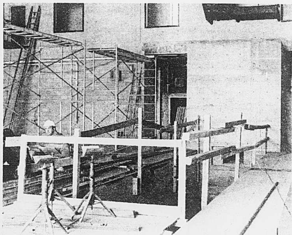
Des véhicules pesant jusqu'à 15,000 livres seront projetés sur ce mur de béton à une vitesse de 30 milles à l'heure.
