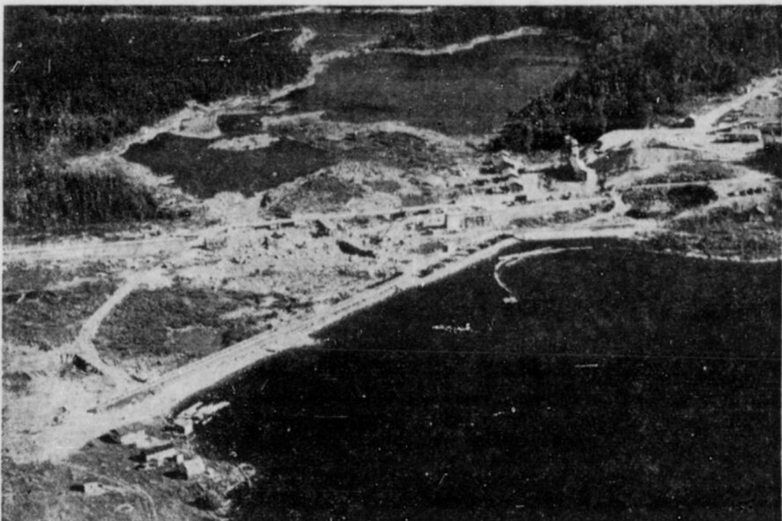
EN PLEINE FORET, 225 hommes construisent le barrage de Cabonga, à la rivière Gens-de-Terre, sous la direction de la firme Dan Lamothe, pour le compte de la commission des ressources hydrauliques, relevant de l'honorable John S. Bourque, ministre des terres et forêts. On y accède par une nouvelle route automobile et le pont Bailey amené de Trois-Rivières. La digue a pour but de régulariser le débit de la Gatineau pour le flottage du bois. Elle aura 1,040 pieds de large. Elle relèvera le niveau de l'eau de 20 pieds, maximum possible, car autrement l'écoulement des eaux se ferait vers le nord.
