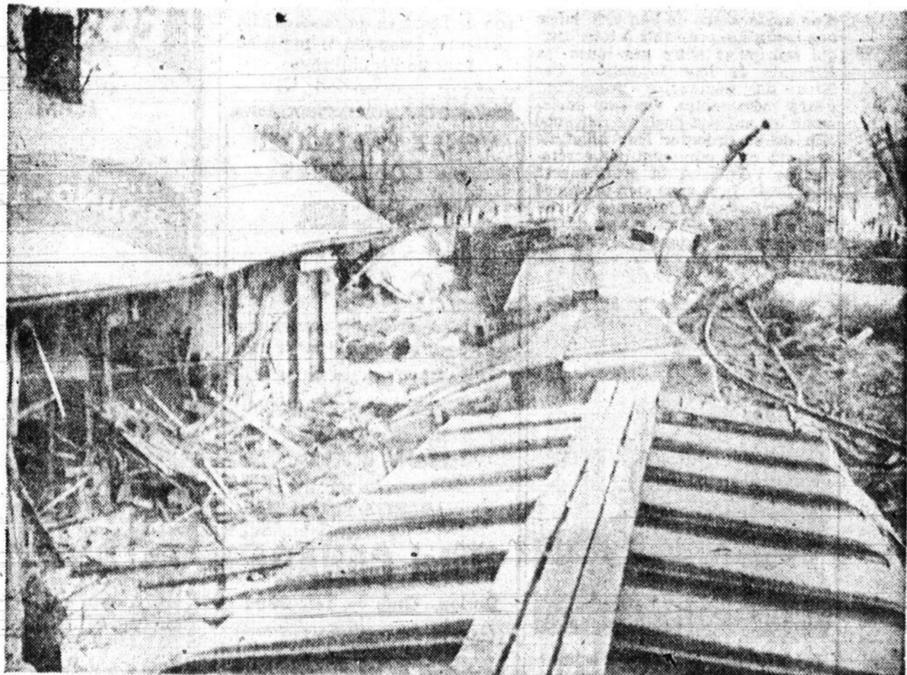
TRENTE WAGONS DERAILLENT — Trente wagons d'un convoi du New York Central ont sauté hors des voies, hier, à Waterloo, dans l'Indiana. Des wagons ont heurté la gare dont la façade a été démolie. Personne n'a perdu la vie dans l'accident. (Fac-similé United Press — "Montréal-Matin")
