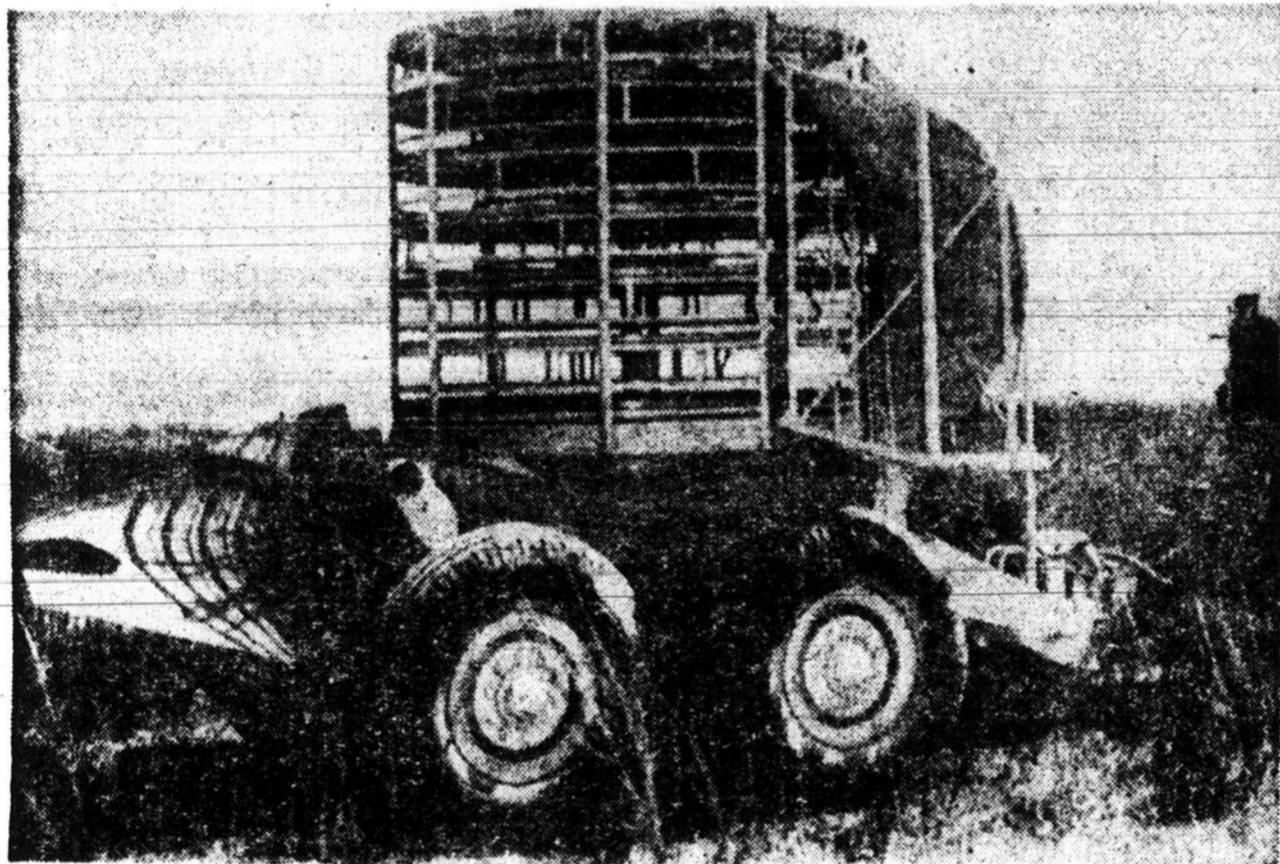
TOUT SE MODERNISE — Il ne s'agit pas d'une machine aratoire... C'est un appareil que vient de créer l'armée américaine et qui, tout en creusant un sillon, "sème" des mines et les recouvre ensuite de terre. (Fac-similé United Press — "Montréal-Matin")
