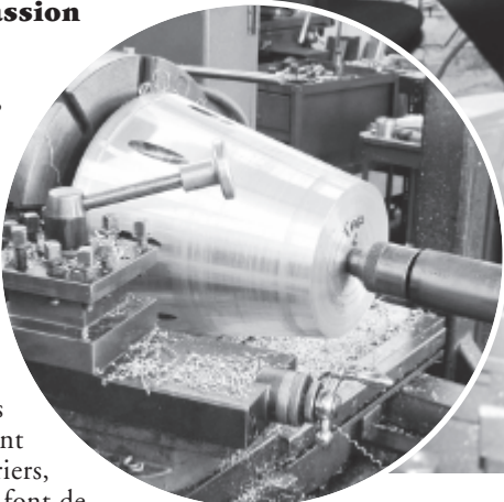
Dans son atelier d'usinage, Wolfgang peut aussi bien réaliser une turbine sophistiquée que refaire une pièce brisée d'un mécanisme. — En mortaise, un tour à métal d'une grande précision.
