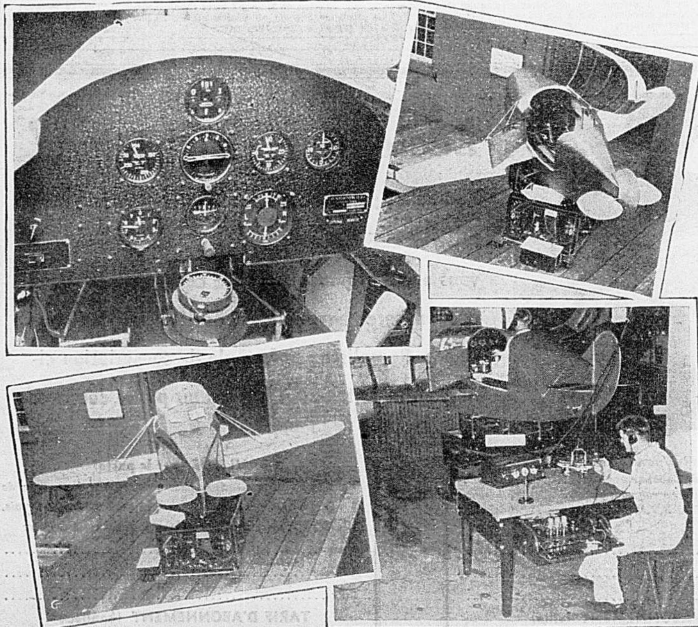
L'on fabrique actuellement à Gananoque, Ontario, un appareil servant à l'entraînement d'aviateurs et ce pour le compte du ministère de l'Aviation britannique. Les photos ci-dessus illustrent les fonctions de l'avion-entraîneur. Au haut à gauche l'on a une vue d'intérieur de la carlingue du pilote avec son tableau de distribution; à droite la carlingue elle-même; au bas à gauche l'avion est prêt à commencer un vol et à droite l'on a un tableau dans lequel tous les mouvements de l'aviateur-écolier sont enregistrés.
