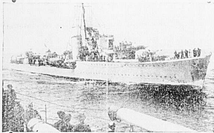
Le "Nestor" (1,690 tonnes) photographié au moment où il apportait des ordres secrets au commandant d'un autre navire de guerre britannique, est un contre-torpilleur de la classe du "Javelin" et il atteint une vitesse de 36 nœuds. C'est un navire de 348 pieds de longueur, armé de six canons de 4,7 pouces, de six pièces de petit calibre et de dix tubes lance-torpilles, de 21 pouces. Plusieurs membres de son équipage de 183 hommes ont été décorés pour la part qu'ils ont prise dans les opérations en Méditerranée.
