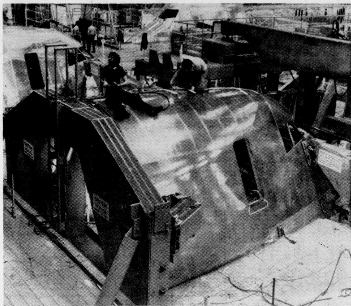
Des ouvriers de Boeing, à Seattle, posent des rivets sur la partie avant du fuselage.
