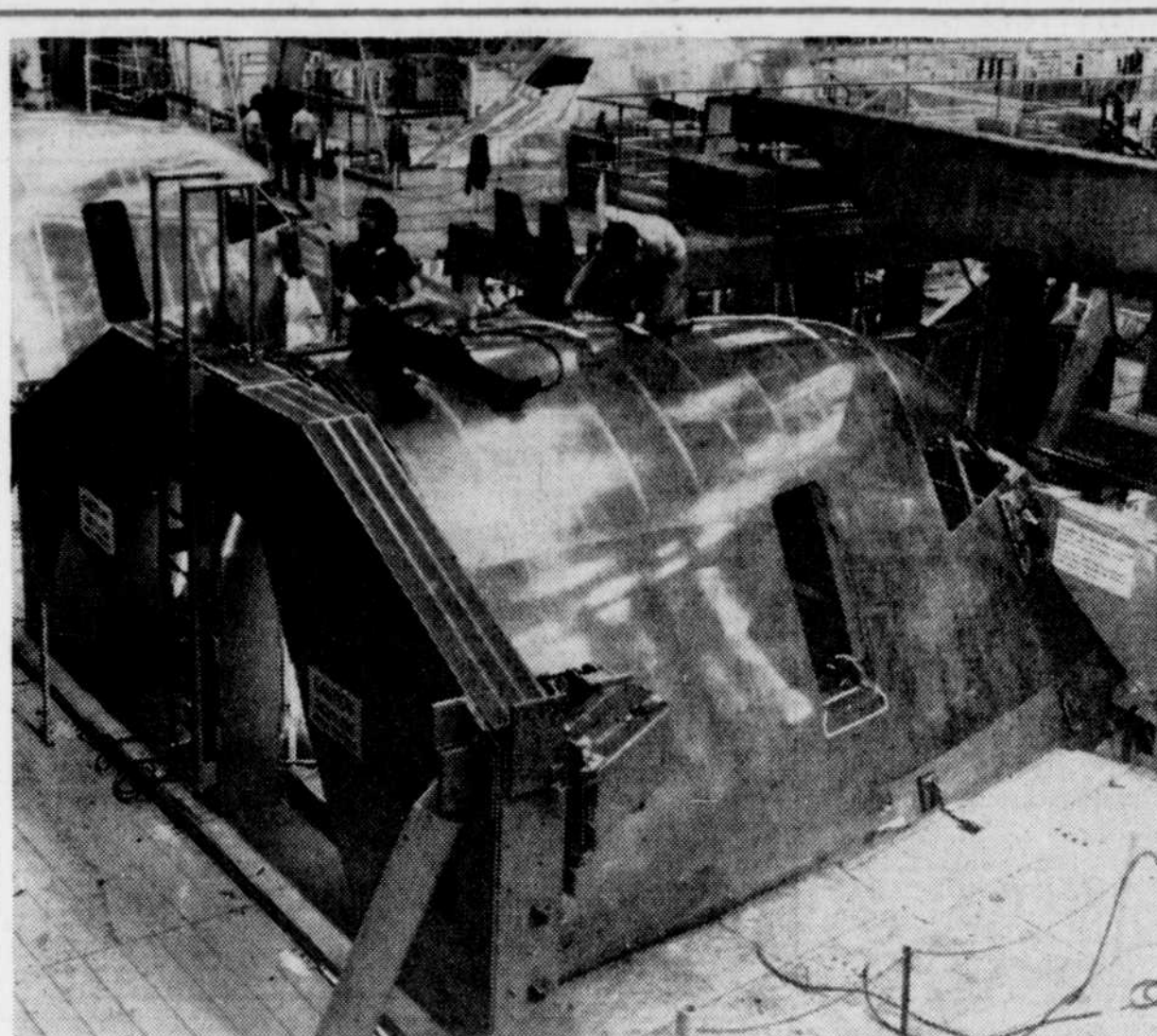
Des ouvriers de Boeing, à Seattle, posent des rivets sur la partie avant du fuselage.
