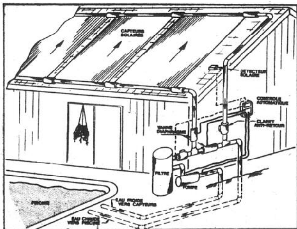
Dessin schématique d'un chauffe-piscine solaire.
