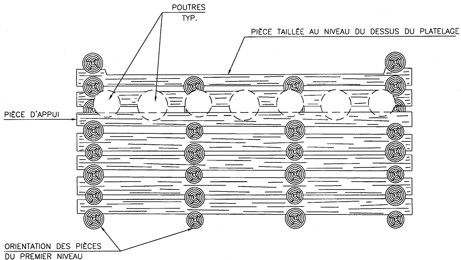
CULÉE (ÉLEVATION AVANT)
