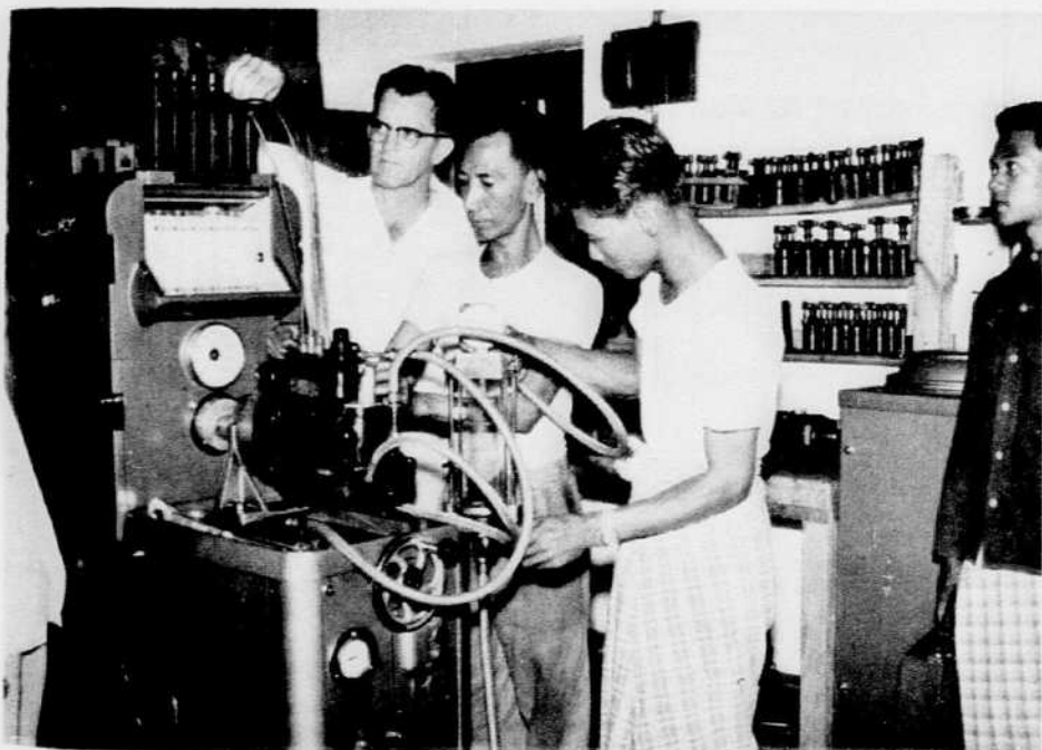
Le Centre d'apprentissage est des mieux équipés. Ici, un expert examine un vérificateur de pompe à carburant pour moteurs diesel. Cette pièce d'équipement du dernier modèle a été obtenue du Canada, grâce au plan Colombo.
