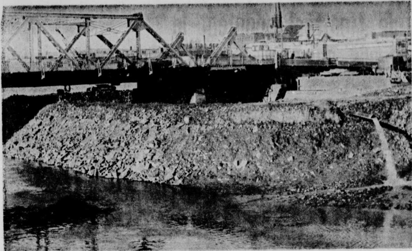
Un batardeau a été édifié à l'extrémité du pont Drouin pour permettre le rejet de l'eau, afin de procéder à l'installation des fondements du futur pont. (Photo : L'Action-Québec, par Marcel Laforce)
