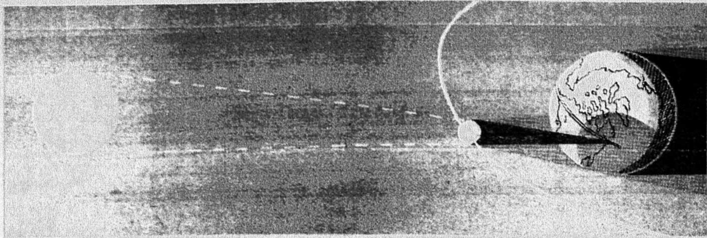
Position relative du soleil, de la lune et de la terre, lors de l'éclipse totale de soleil le 20 juillet prochain. Le sentier d'éclipse totale, cheminant depuis le Japon jusqu'à l'océan Atlantique, en passant par l'Alaska et le Québec, n'aura qu'une largeur de 55 à 60 milles. Un vaste secteur de l'Amérique du Nord et de l'Amérique Centrale sera plongé dans la pénombre, indiquée ici en demi-teinte.
