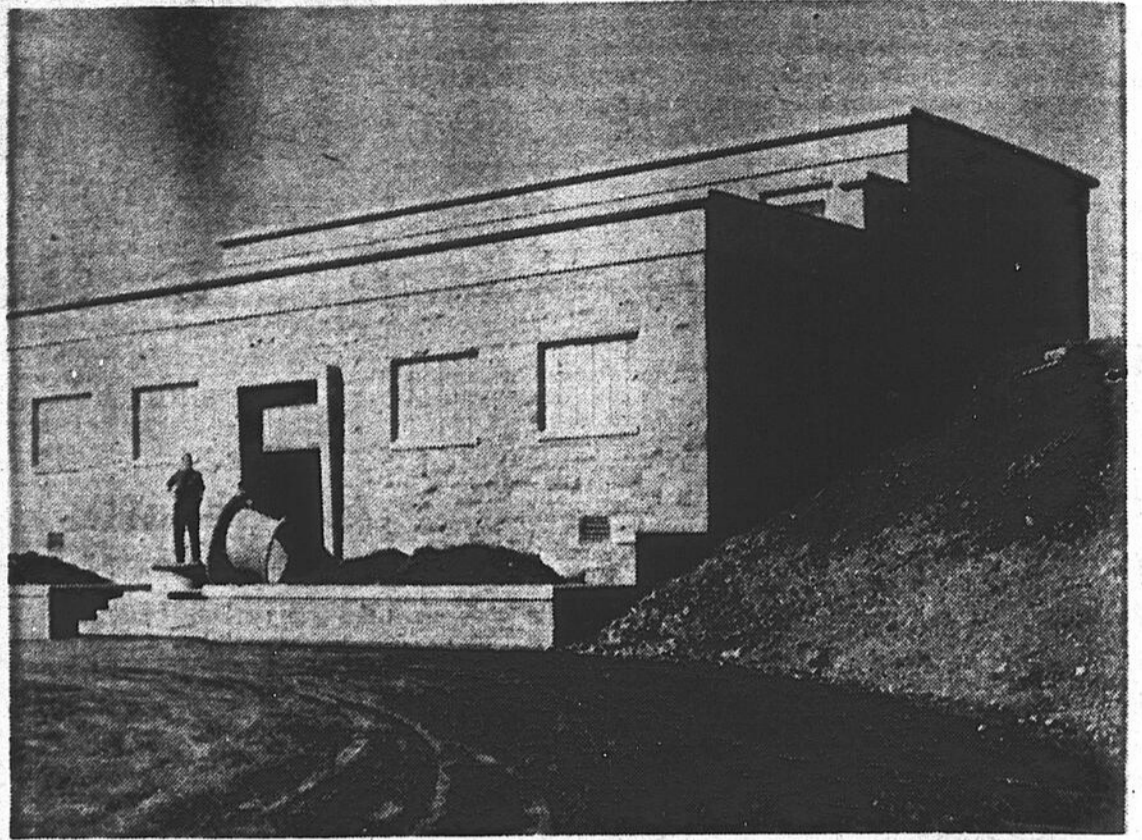
LA CHAMBRE DE CONTROLE DU RESERVOIR — La chambre de contrôle du réservoir de Rosemont est située sur la 16e Avenue. Aboutit à cette endroit la conduite Bourbonnière, qui amène l'eau de l'usine de filtration de l'aqueduc. La chambre abrite des vannes qui permettent de contrôler la quantité d'eau contenue dans les deux cellules du réservoir. Celui-ci sera mis en service au cours du mois de mars.
