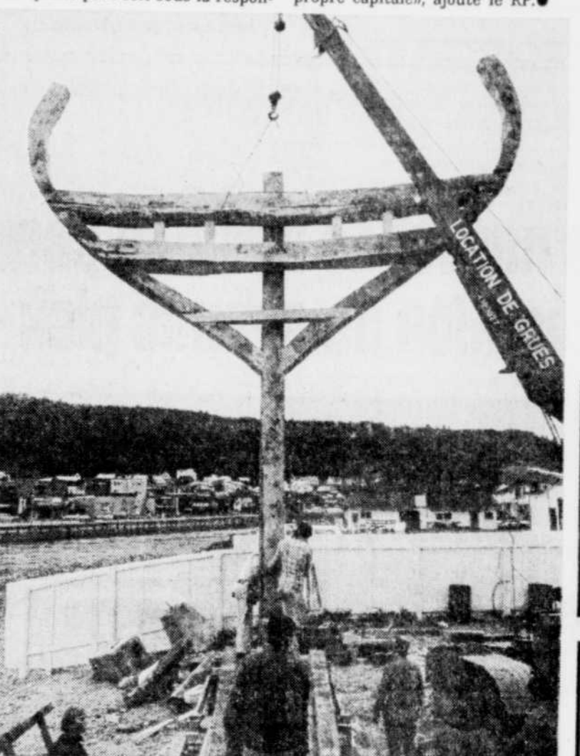
Le tableau arrière qui a 24 pieds de hauteur a été réuni à la quille, hier matin. La pièce de plus de 4 tonnes qu'il a fallu élever avec une grue y est attachée par un talon de bois.
