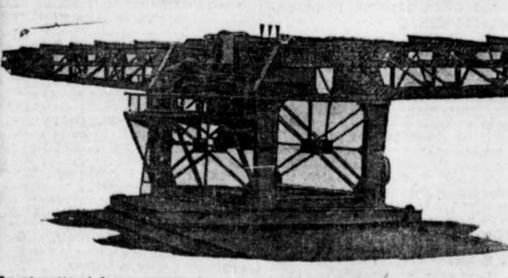
La vignette ci-dessus montre la grue qui vient de faire ses premiers essais, samedi dernier, aux hangars du Pacifique. On peut se rendre compte de la puissance formidable de cet appareil et de ses dimensions. A droite et en bas de la gravure, on aperçoit le mécanisme qui sert au fonctionnement de la machine.
