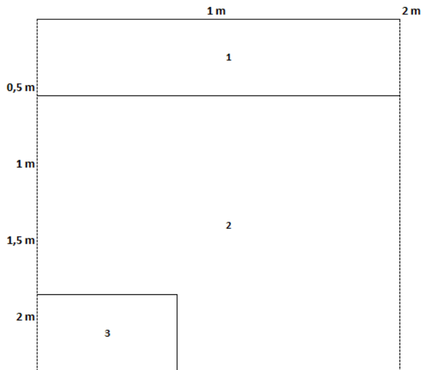
Figure 15. Croquis stratigraphique C2
