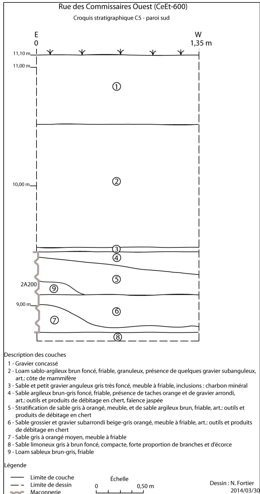
Figure 17. Croquis stratigraphique C5
