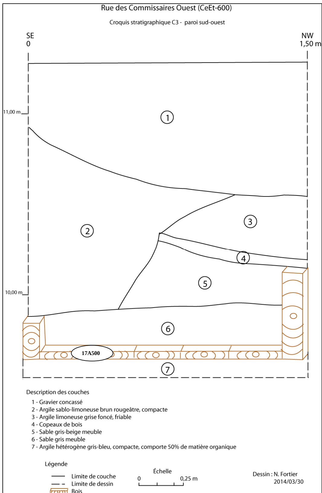
Figure 19. Croquis stratigraphique C3
