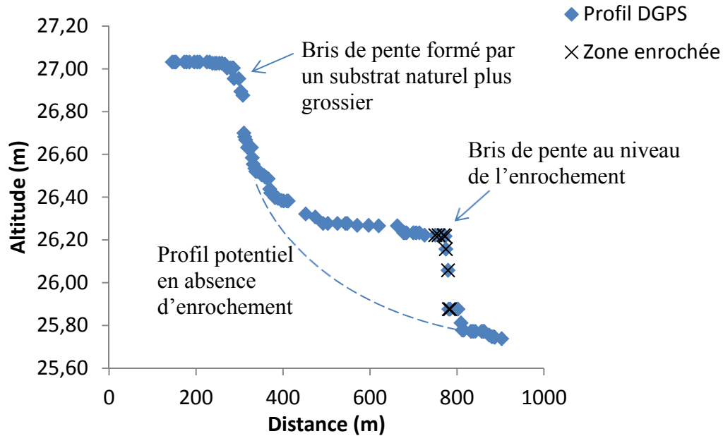
Figure 6 Exemple de profil longitudinal de la surface de l'eau (pont 17399)
