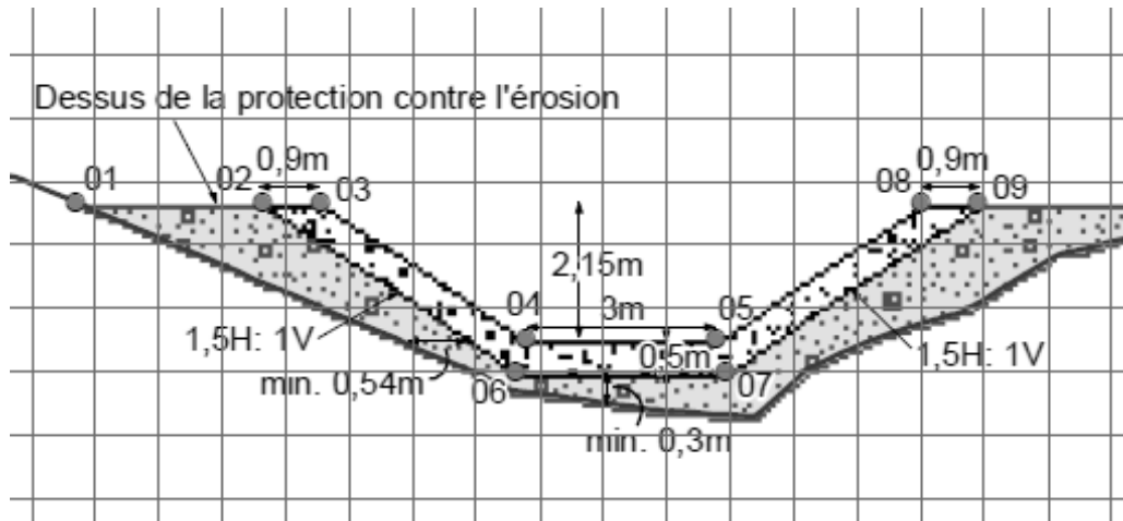
Figure 13 Plan d'une coupe transversale de l'enrochement sur le tributaire 5 de la rivière Salvail
