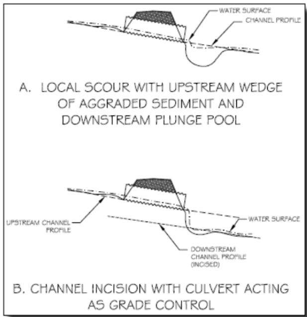
Figure 7 Aggradation due à un refoulement en amont d'une structure accompagnée d'un affouillement (A) ou d'une incision (B) sur un cours d'eau en aval (USDA 2008).
