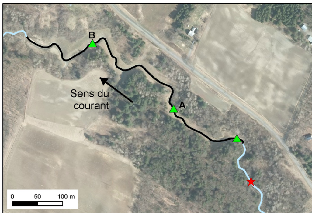
Figure 15 Localisation des installations sur le tributaire 5 de la rivière Salvail La zone enrochée est représentée en noir. Les triangles verts représentent les sondes mesurant la surface de l'eau, avec en plus des piézomètres aux points A et B. L'étoile rouge représente le barrage à encoche en V mesurant le débit (voir Figure 17).
