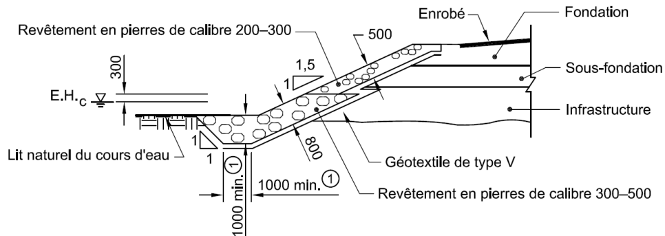
Figure 2 Plan en coupe d'un enrochement typique.
