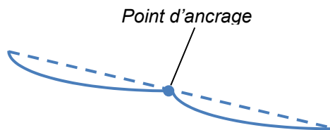
Figure 9 Évolution schématisée d'un profil non à l'équilibre (en tiretés) vers un profil à l'équilibre (en bleu continue) en présence d'un point d'ancrage (« grade control point »).
