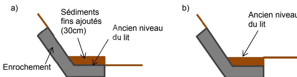
Figure 11 Schéma des enrochements réalisés sur la rivière Richelieu en 2013 (a) et en 2014 (b)
