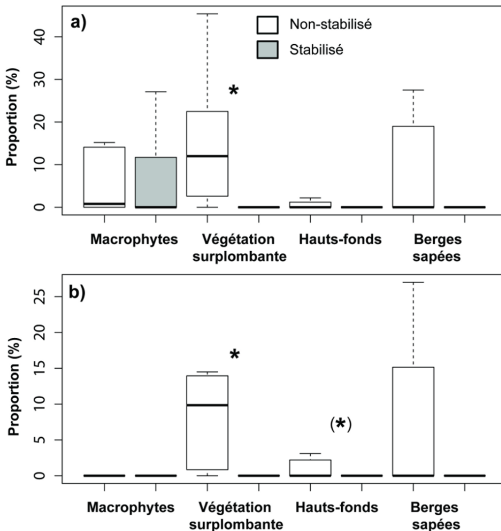
Figure 25 Proportions des différents types d'abris dans les Basses-Terres (a) et dans les Appalaches (b) pour les sites enrochés et non enrochés
