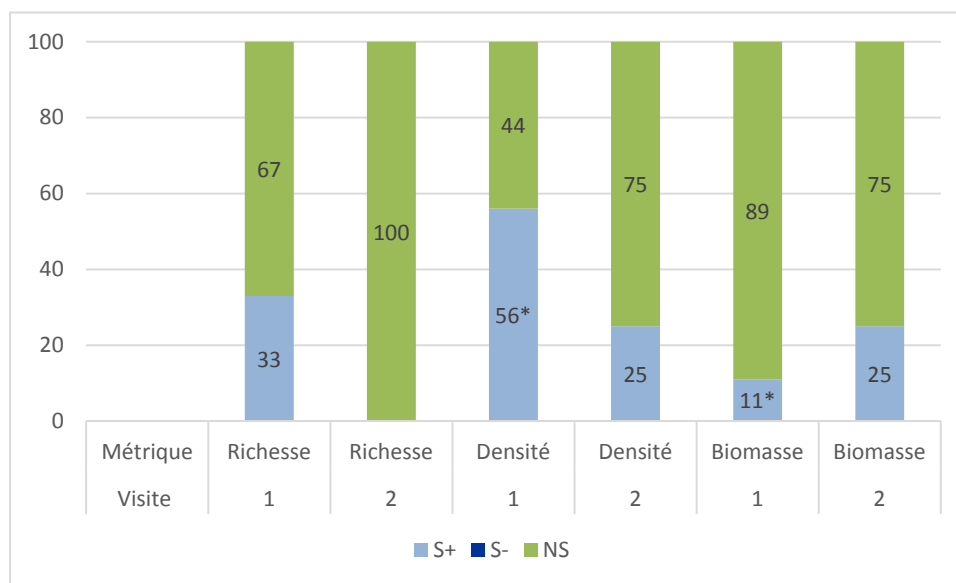
Figure 32 Résultats des différents tests T de Student (en %) effectués pour chacune des métriques de poissons et pour chacune des visites S+ représente les tests significativement positifs, S- les tests significativement négatifs et NS les résultats non significatifs. * Indique la significativité du test de Fisher.
