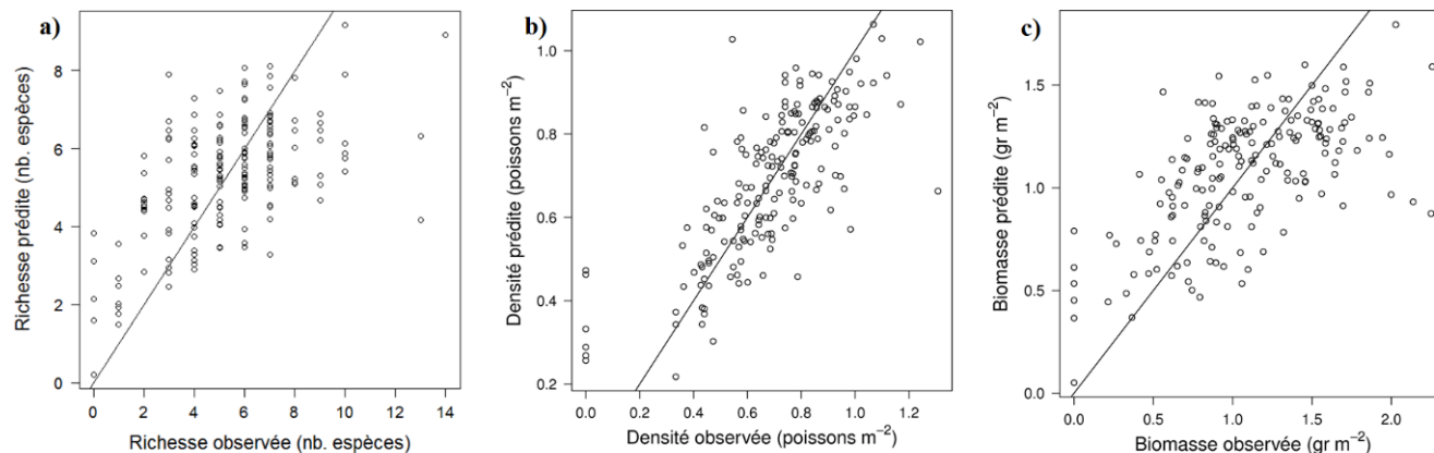
Figure 33 Modèles prédictifs pour les trois métriques de poissons, soit les valeurs prédites en fonction des valeurs observées pour a) la richesse, b) la densité et c) la biomasse Une ligne représentant une relation 1 : 1 est superposée au graphique.
