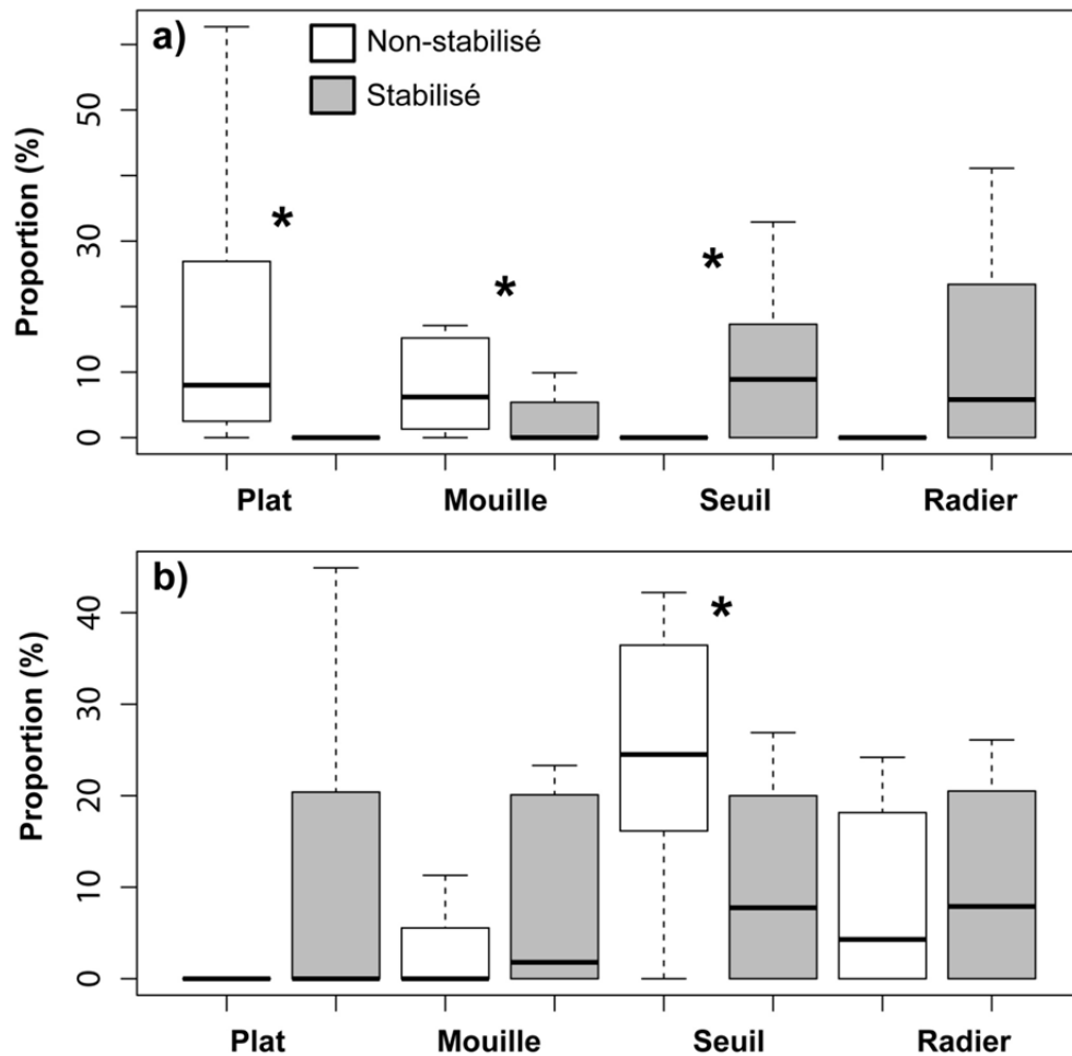
Figure 24 Proportions des mésohabitats dans les Basses-Terres (a) et les Appalaches (b) pour les sites enrochés et non enrochés L'astérisque indique une différence de moyenne significative ( p < 0.05 ). La proportion de radier dans les Basses-Terres étant de 0%, ce cas n'a pas été testé statistiquement.
