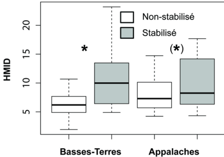
Figure 26 Scores HMID dans les Basses-Terres et les Appalaches aux sites enrochés et non enrochés
