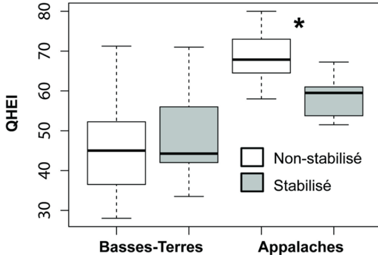
Figure 27 Scores QHEI dans les Basses-Terres et les Appalaches aux sites enrochés et non enrochés L'astérisque indique une différence de moyenne significative ( p < 0.05 ).
