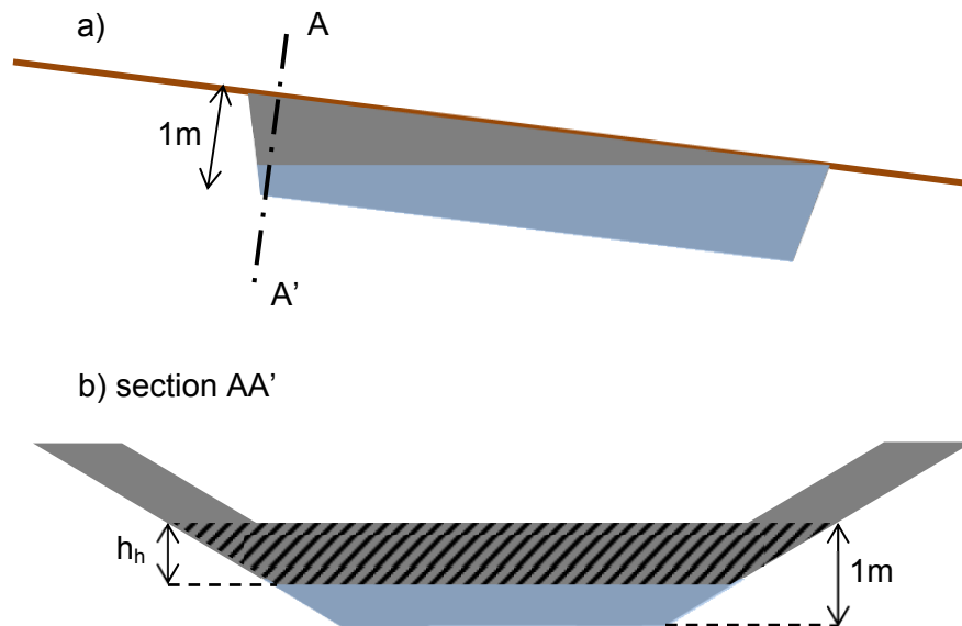
Figure 18 Schéma des écoulements hyporhéiques dans un enrochement Sur le profil longitudinal (a), une zone de refoulement (en bleu) apparaît dans l'enrochement (en gris). La zone d'écoulement hyporhéique maximale se situe à la section transversale AA' (zone hachurée de hauteur h_h , figure b), au-dessus de la zone de refoulement.
