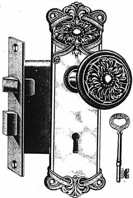
No 651-050. - Modèle "Concord." Fer fondu, plaqué vieux cuivre. Pour serrures de portes de façade et de portes intérieures.
