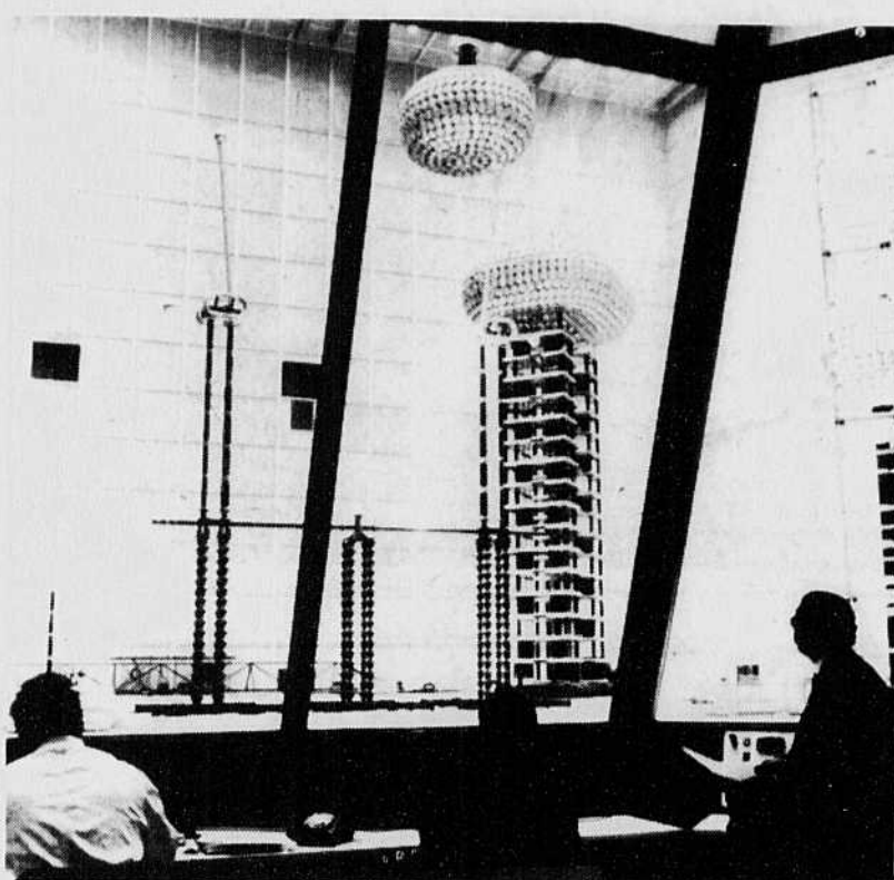
Des experts testent des équipements de transmission à haute tension dans un laboratoire d'Hydro-Québec. En 1991, bien que les Québécois vivent sous quelque 120 000 kilomètres de lignes électriques, le milieu scientifique dispose de très peu d'informations sûres concernant les effets biologiques des champs électriques et magnétiques sur la santé.
