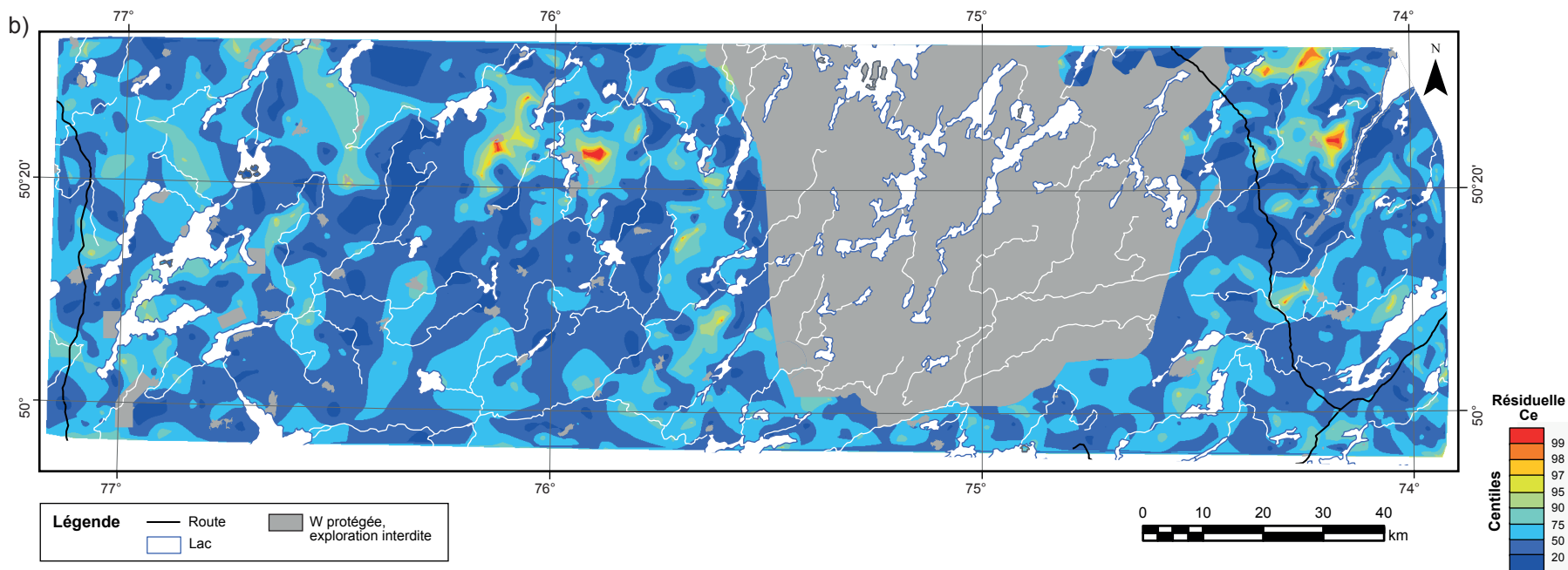
FIGURE 4 – a) Carte des concentrations en Ce dans les sédiments de fond de lac du levé Assinica. b) Carte des valeurs résiduelles après traitement de régression spatiale pour le cérium.
