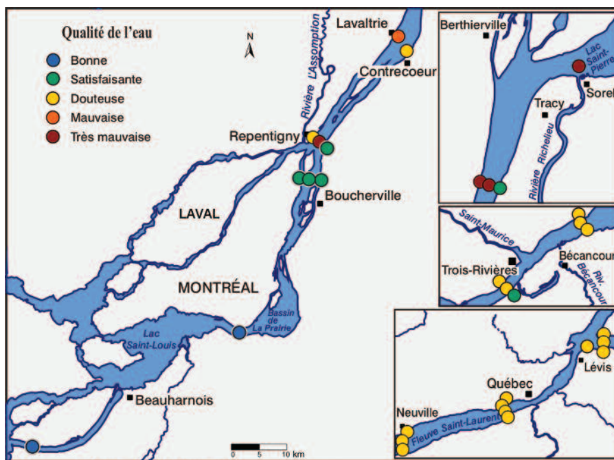
FIGURE 3. QUALITÉ DE L'EAU DU FLEUVE SAINT-LAURENT, ÉTÉS 2004 ET 2005
