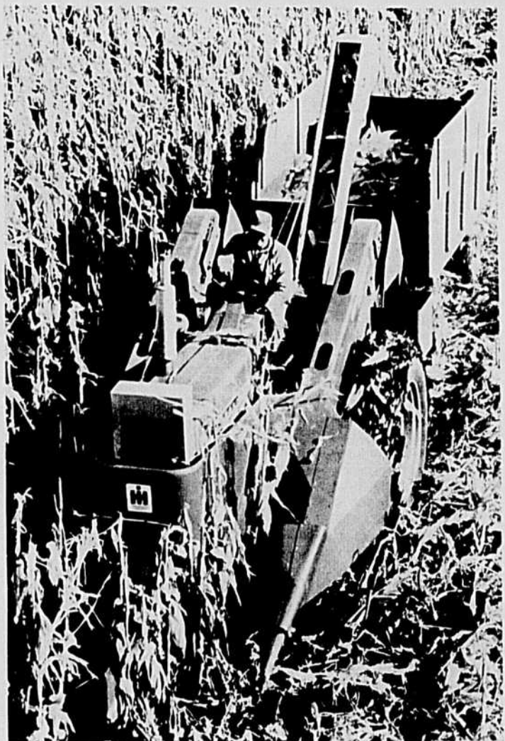
Le nouveau IH 234 Corn Harvester. Une possibilité d'adaptation universelle pour 26 modèles différents de six fabrications de tracteurs. Le 234 prévoit toute l'économie efficace d'une tête combinée à maïs plus la versatilité des changements arrière d'unités
