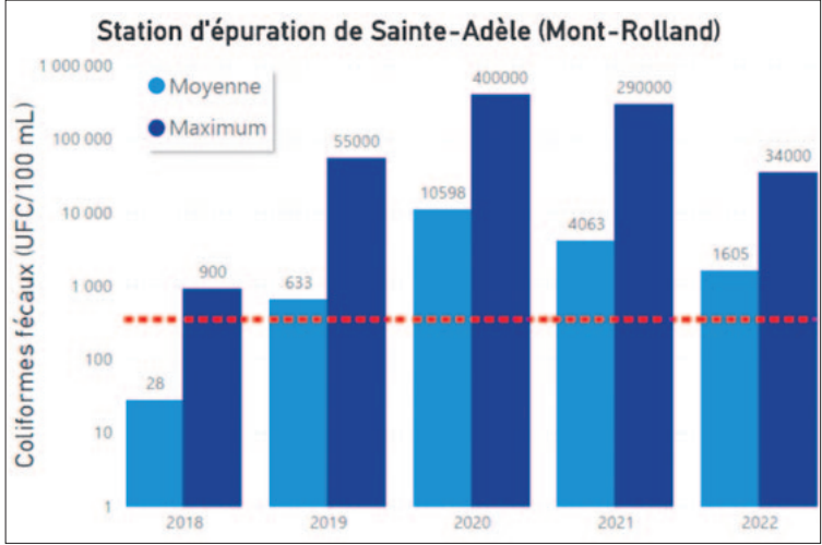
Moyennes géométriques et valeurs maximales de concentration en coliformes fécaux à l'effluent de la station d'épuration de Sainte-Adèle (Mont-Rolland) en période estivale (juin à septembre) entre 2018 et 2022. La ligne rouge pointillée correspond à la norme supplémentaire de rejet en coliformes fécaux de 350 UFC/100 ml (moyenne géométrique calculée sur une base mensuelle)
