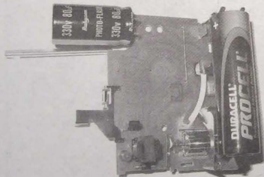
La fameuse carte contenant le condensateur du flash de notre appareil photo jetable après mise en pièce
