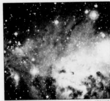
Un coin de notre Voie lactée.
