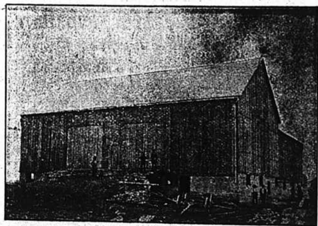
Grange de Allan McMane, Atwood, Ont. Dimensions des murs: 84 x 100 x 9 pieds de haut. Construits avec le CIMENT THOROLD en 1898.
