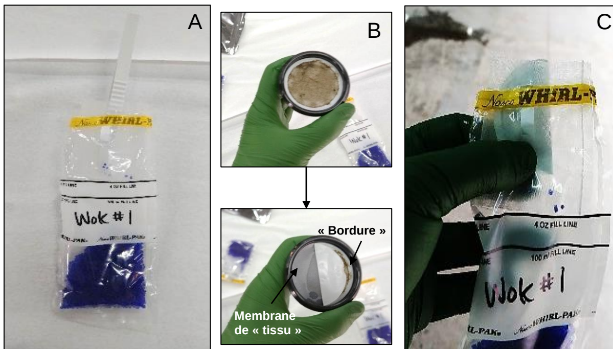
Figure 15. A) Sac Whirl-PAK MC avec des billes de silice; B) Retrait et pliage du filtre avec une pince; C) Disposition du filtre dans une pochette de nylon, dans le sac Whirl-PAK MC
