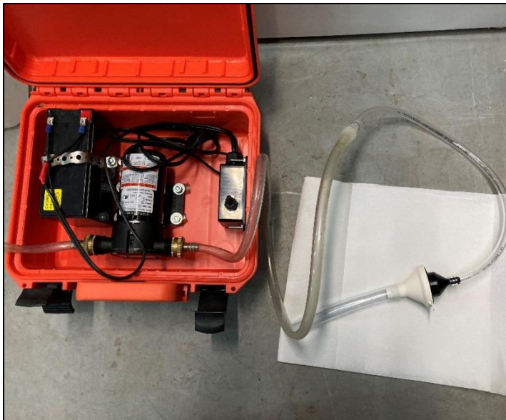
Figure 13. Installation lors de la filtration d'un échantillon d'eau
