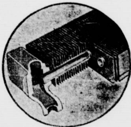
COUPE DU NOUVEL ELEMENT ROSEMOUNT
