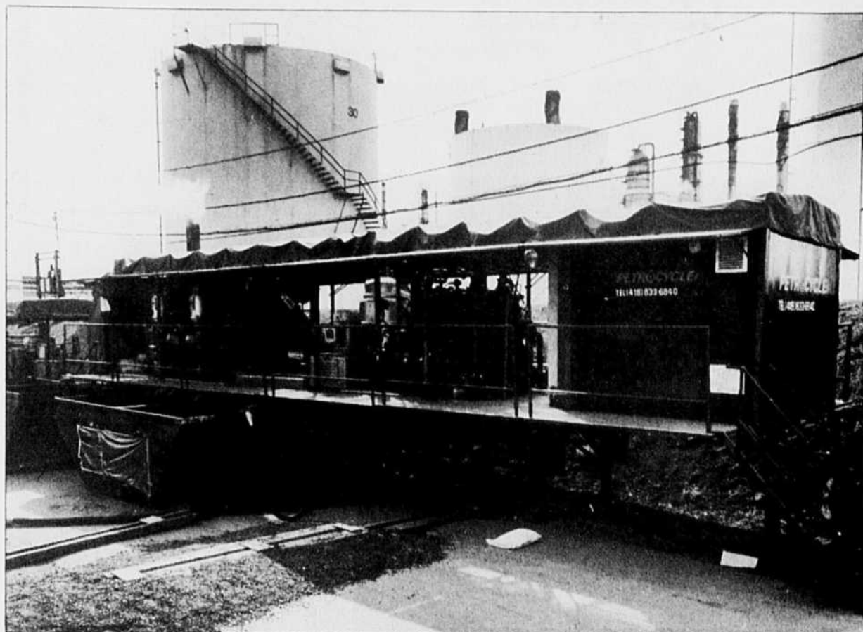
Cette centrifugeuse française permet de récupérer sous forme d'huile environ 70 % des résidus d'hydrocarbures que les raffineurs entreposent dans des réservoirs comme ceux que l'on voit derrière. Il existe environ 75,000 tonnes de résidus de raffinage entreposés à travers le pays.
