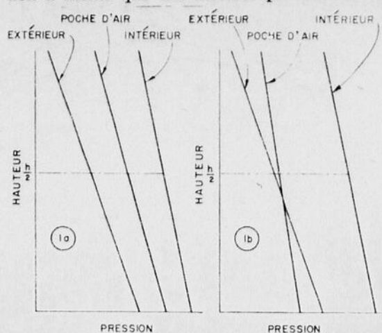
FIGURE 1 RÉPARTITION DES PRESSIONS AU TRAVERS DE FENÊTRES DOUBLES, L'AIR S'ÉCOULANT DE L'INTÉRIEUR VERS L'EXTÉRIEUR.
