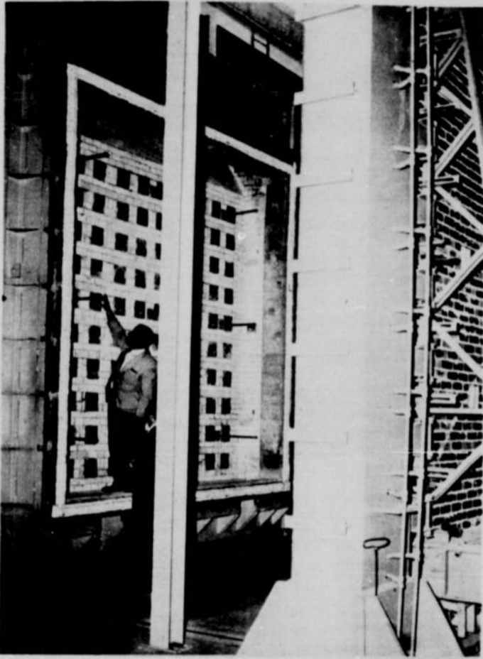
△ Le puissant four, unique au Canada, constitué de cent bouches à feu utilisé au Laboratoire du Feu pour l'étude de la résistance des murs de brique (à l'extrême droite) ou autres à la chaleur et aux flammes. Les jets de gaz enflammés sont projetés contre le mur pendant un certain nombre d'heures et des appareils enregistrent tout ce qui se passe.
