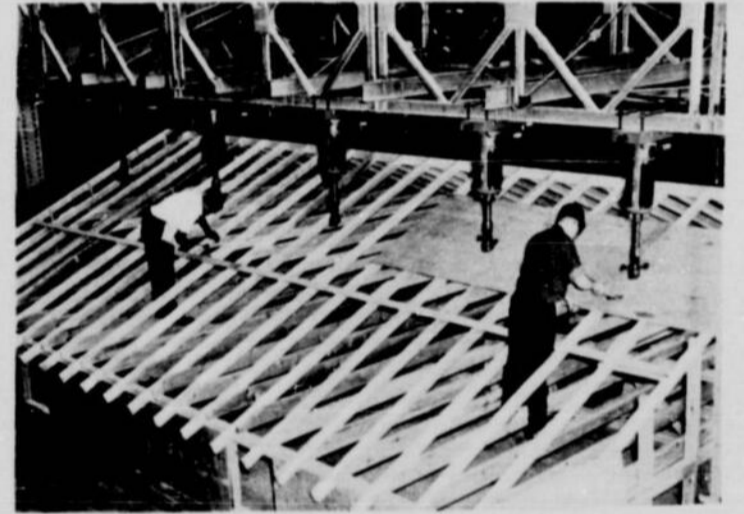
△ Construction en laboratoire d'une toiture entière et véritable de maison que les tiges d'acier fixées à la superstructure mobile surplombant le toit viendront écraser ensuite sous une pression scientifiquement déterminée d'avance pour étudier la résistance des matériaux de construction.
