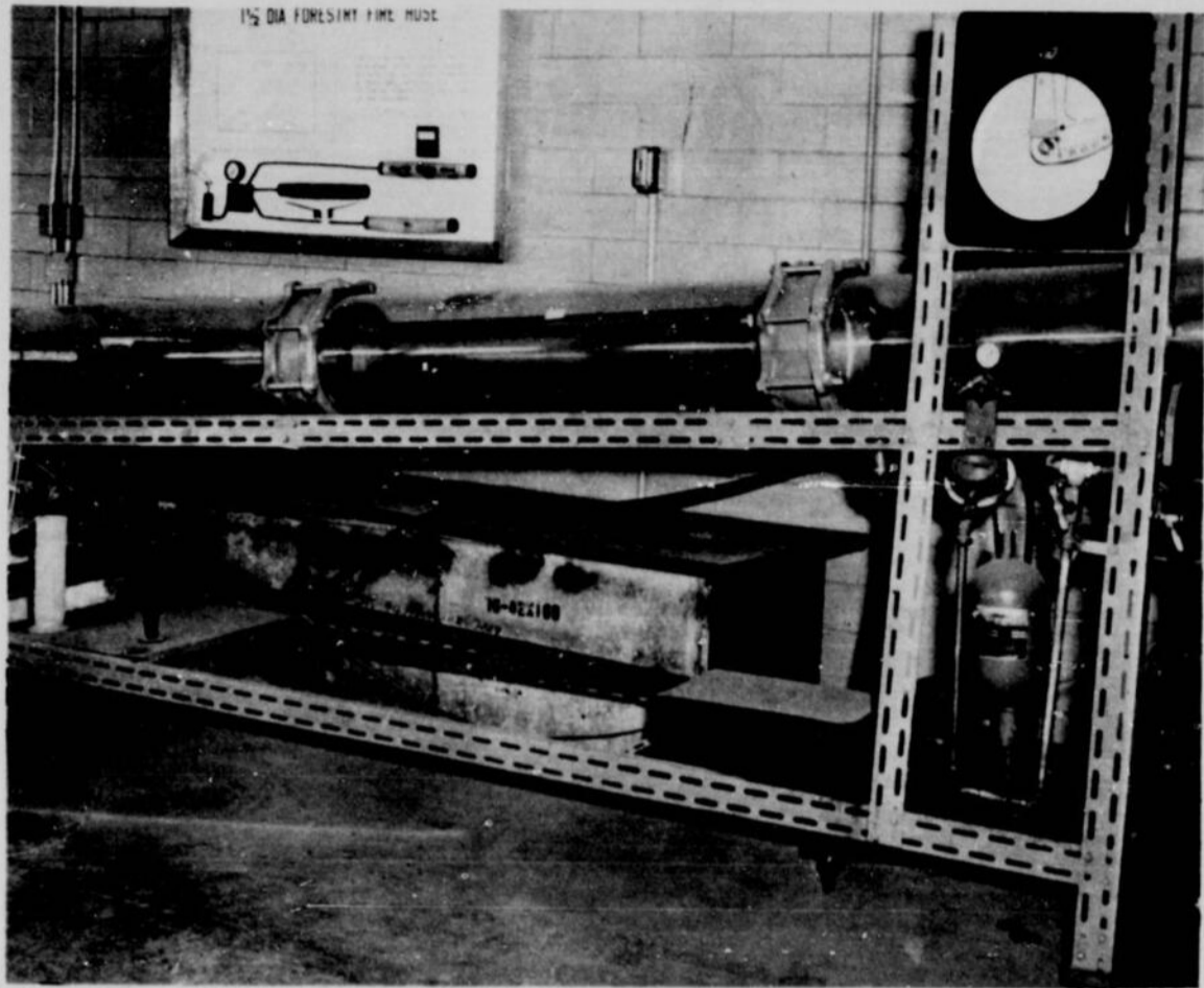
△ Voilà un appareil bien curieux. Il sert à étudier l'effet du feu ou des flammèches atteignant des boyaux d'arrosage de divers types utilisés dans la lutte contre les feux de forêt pour voir quelle est leur pouvoir de résistance au feu.
