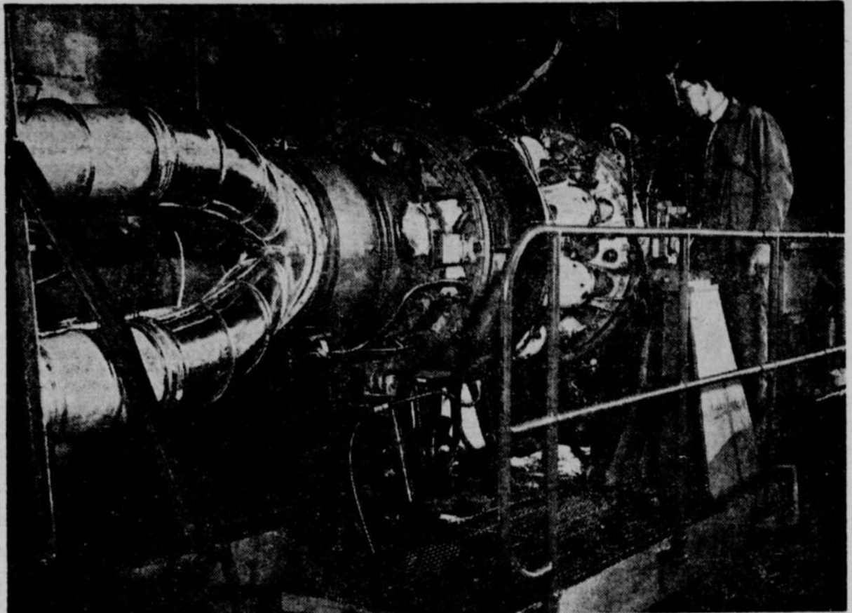
VOICI LE MOTEUR DU "BLUEBIRD", la voiture avec laquelle Donald Campbell tentera d'atteindre une vitesse de 400 milles à l'heure cette semaine à Bonneville, Utah. Le moteur est un modèle Proteus, fabriqué par Bristol-Siddeley, et est aussi employé dans les avions Britannia.
