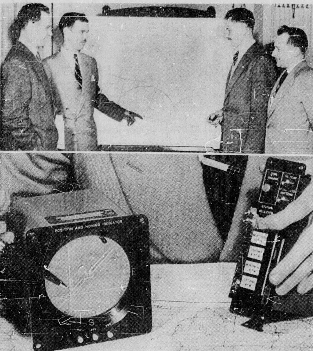
NAVIGATION AERIEENNE AUTOMATIQUE—Une entreprise d'Ottawa, Computing Devices of Canada, vient de réaliser les plans d'un instrument de navigation aérienne à bouton-pression unique en son genre et procédé à sa fabrication. Spécialement destiné aux chasseurs à réaction du C.A.R.C., l'appareil remplace à la fois les cartes de navigation et la boussole. Il est l'invention de M. J. Stuart Parsons, ingénieur-chef de Computing Devices of Canada, chemin Richmond. Nous voyons, de gauche à droite sur la photo, M. B. Halford, M. Parsons, M. H. C. Luttman, M. J.-P. Duhamel, ingénieur en électricité, collaborateur de M. Parsons, nouveau de M. Charles Gauthier, autrefois rédacteur en chef au "Droit" et de M. Roméo Duhamel, typographe à notre journal. MM. Halford et Luttman étaient deux visiteurs invités de la compagnie. Au nombre des directeurs présents, mentionnons le contre-amiral G. I. Stephens, C.B., C.B.E., M.R.C., (à sa retraite), récemment nommé directeur. Il habite Ottawa depuis 1941. Nous remarquons en bas, les boutons-pression et l'écran, parties visibles de l'appareil dans la cabine du pilote d'avion à réaction. (Photo "Le Droit"—par Champlain Marcell)
