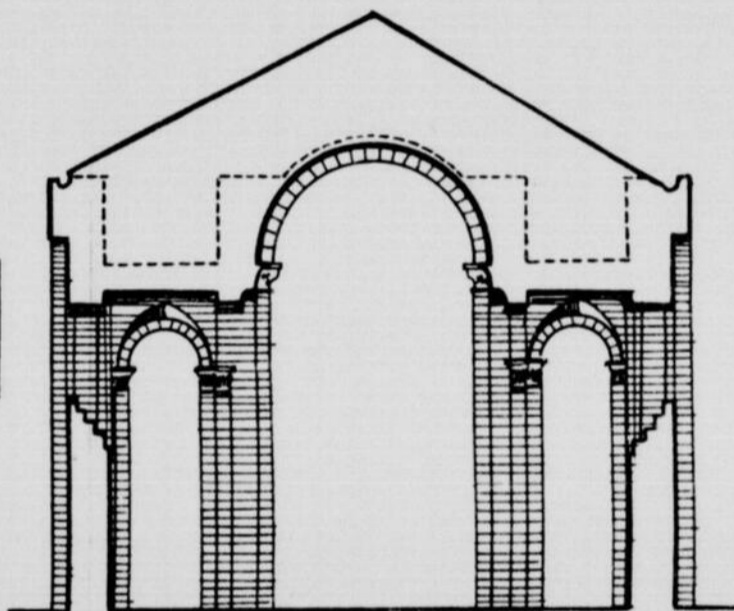
PLAN ET COUPE D'UNE ÉGLISE ROMANE
