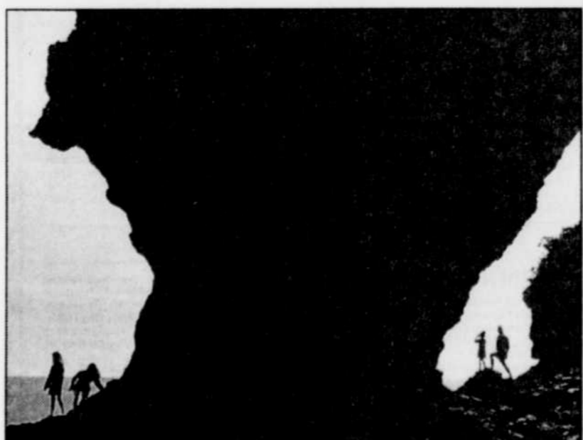
Les «demoiselles» de Hopewell (N.-B.). À marée haute, ces formations géologiques redeviendront des îles.
