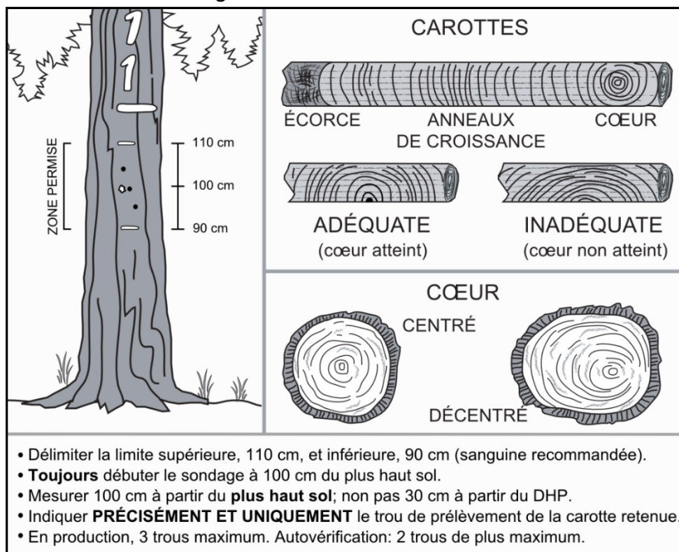
Figure 57 Prélèvement de carottes
