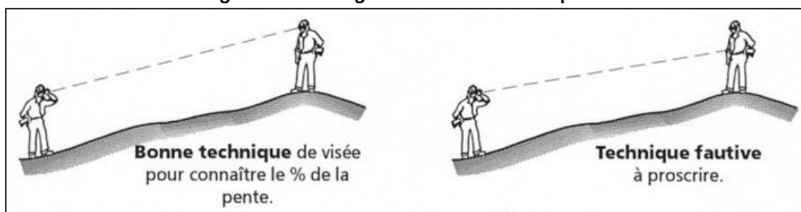
Figure 67 Mesurage de l'inclinaison de la pente
