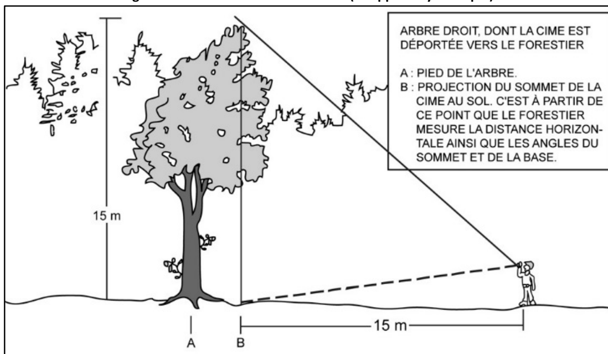
Figure 55 Mesure de hauteur d'arbre (houppier asymétrique)
