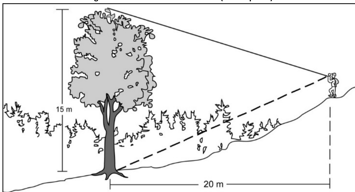
Figure 56 Mesure de hauteur d'arbre (terrain pentu)
