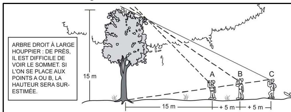
Figure 54 Mesure de hauteur d'arbre
