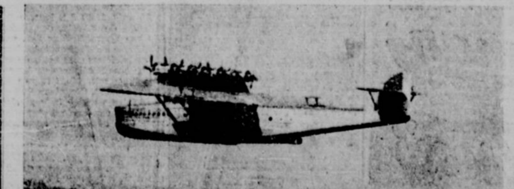
Photo prise pendant l'envolée d'essai de l'avion géant «Dornier», qui a été construit secrètement en Allemagne. Bien que huit de ses douze moteurs seulement fussent utilisés, le géant de l'air s'est élevé avec grâce au-dessus des eaux du Lac Constance, en Suisse, jusqu'à une hauteur de 600 pieds.
