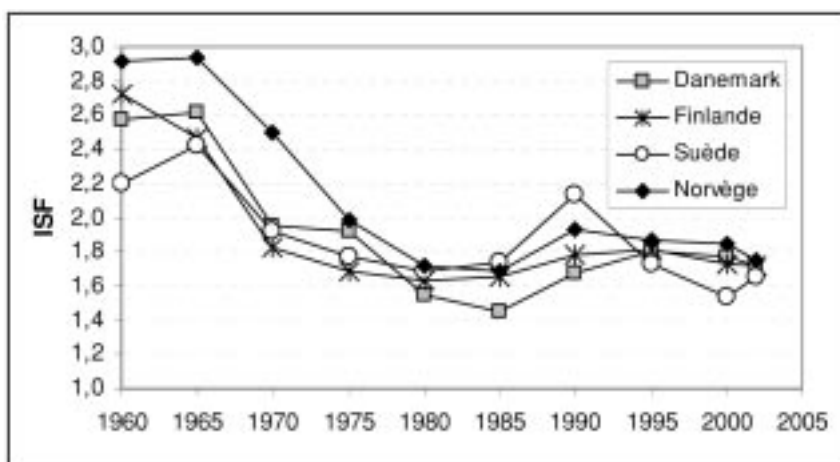
Figure 3 Évolution de l'indice synthétique de fécondité, pays nordiques, 1960-2002
