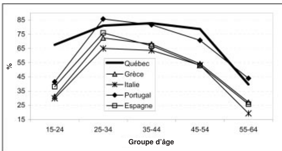
Figure 35 Taux d'activité des femmes, selon le groupe d'âge, Québec et pays de l'Europe du Sud, 2003
