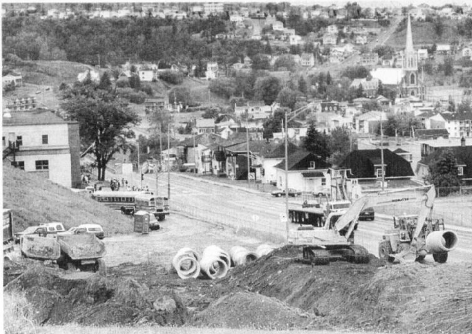
CHANTIER - Les automobilistes circulant sur le boulevard de l'Université, à Chicoutimi, à la hauteur du Parc Jean-Béliveau, sont témoins, ces jours-ci, d'activités de construction spectaculaires. Il s'agit de travaux menés par la Société québécoise d'assainissement des eaux qui aménage le régulateur Bégin. Ces travaux devaient se réaliser après la mise en marche de l'usine d'épuration de la ville. Des changements impressionnants. (Photo Rocket Lavoie)
