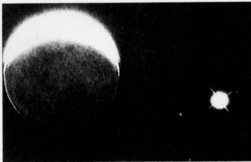
Vénus, telle que vous pouvez la voir en début de soirée au-dessus de l'horizon sud-ouest, pas tellement loin du croissant lunaire (ci-dessus), et telle que photographiée par la sonde américaine Magellan en 1991 (ci-contre).
