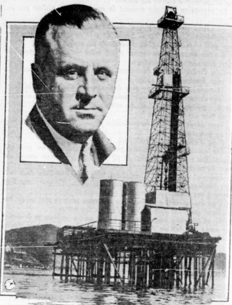
L'île d'acier pour l'embarquement du pétrole, à Ventura, Californie. Dans le médaillon, l'ingénieur C. L. Roberts, qui en eut l'idée et la construisit.
