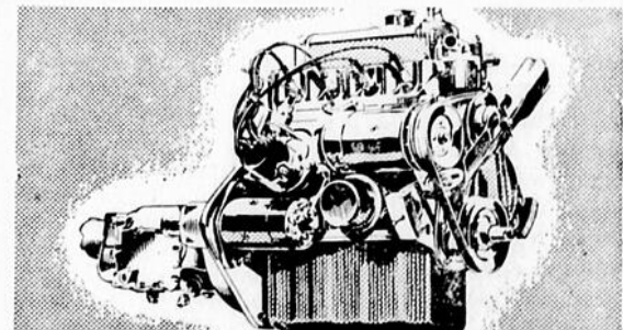
Le nouveau moteur à soupapes en tête ayant servi au test. Toutes les nouvelles Morris Minor sont munies de ce nouveau moteur à 4 cylindres. Le contrôleur de mélange et la pipe d'admission (throttle) sont coordonnés, ce qui permet des démarrages plus rapides, même par les temps les plus froids.
