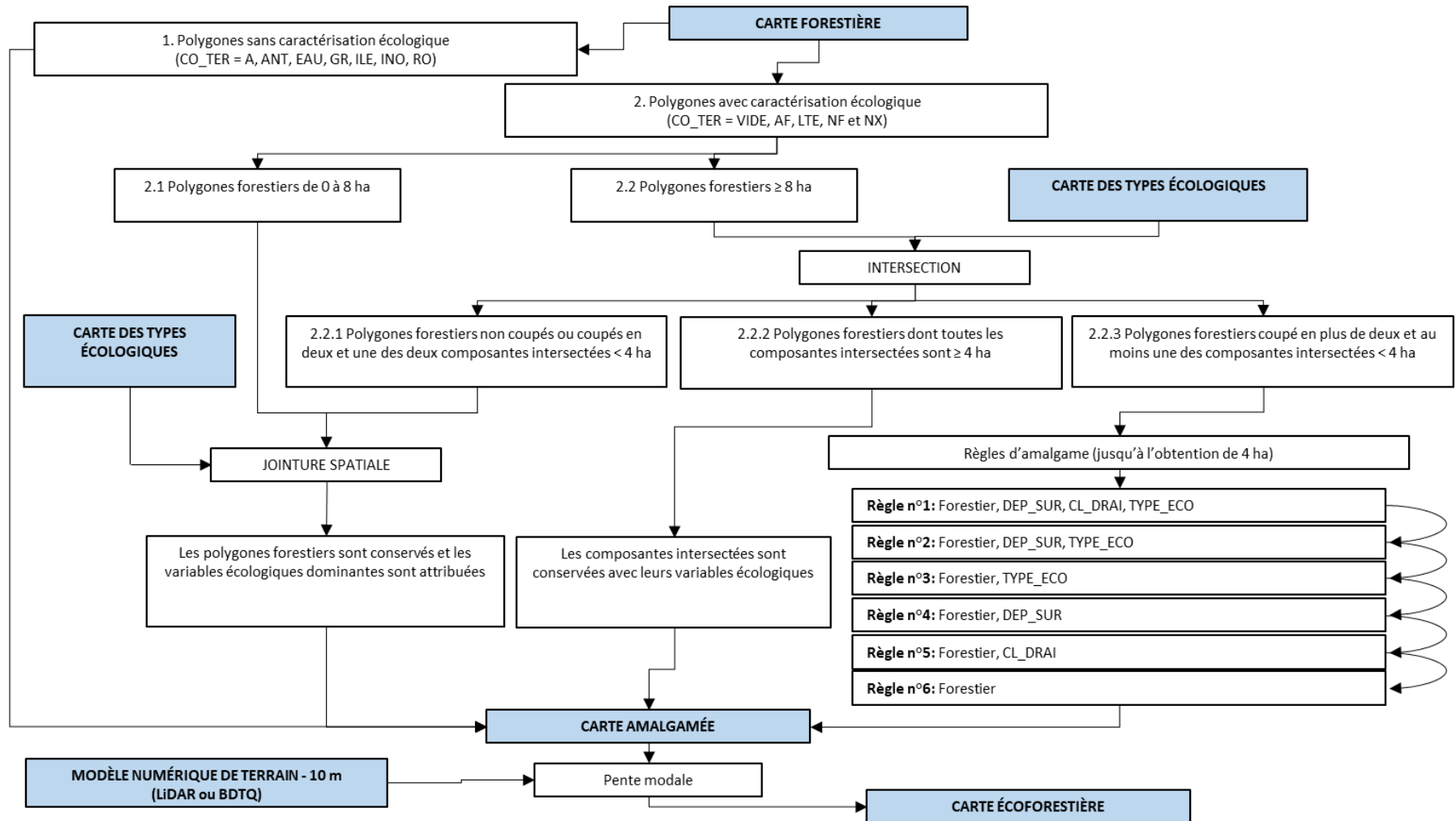
Figure 19. Fonctionnement de l'outil d'amalgame
