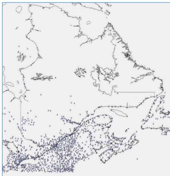
Figure 20. Localisation des stations météorologiques de 1981 à 2010 pour l'ensemble de la province
