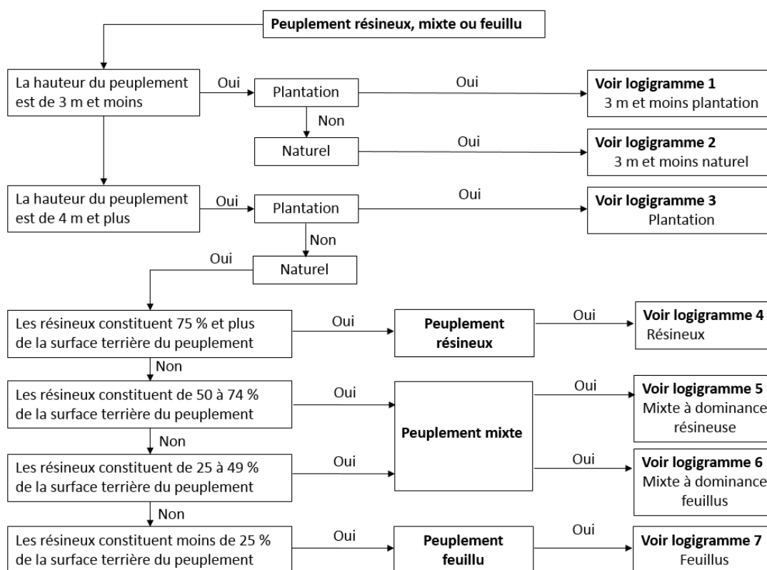
Figure 7. Ordre de priorité des groupements d'essences
