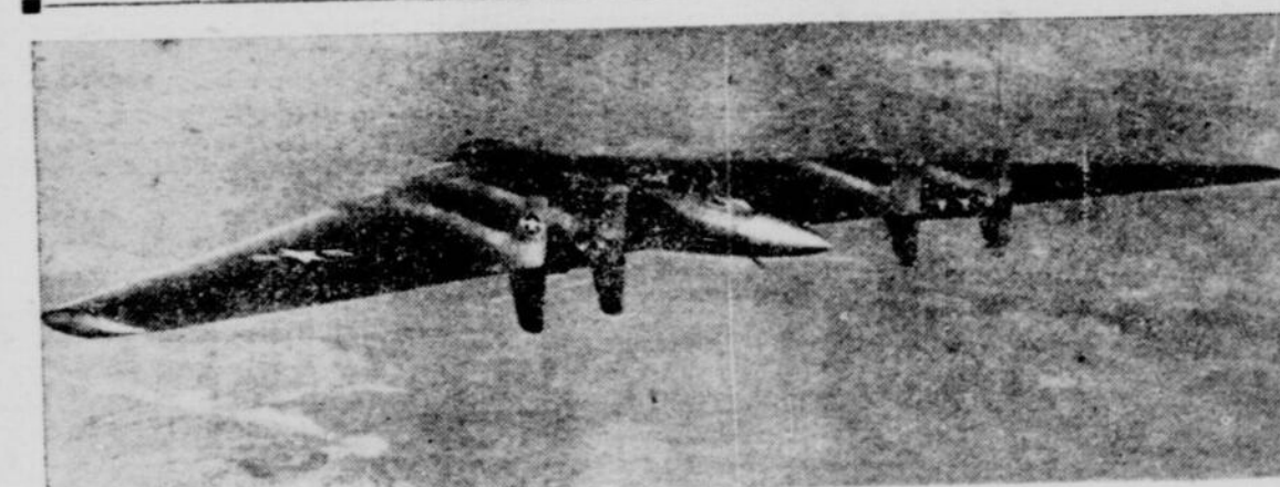
Cette "aile volante" est le plus puissant avion réacté au monde. On en fait l'essai dans le ciel du désert californien. Il est formé d'une aile, à cabine centrale, réservoirs empennés, gouvernails et palonniers au taillant antérieur. Chaque moteur a deux lances, dont les jets fournissent 32,000 chevaux-vapeur. Le monstre peut porter 15 tonnes de bombes, à une vitesse de 500 milles à l'heure.
